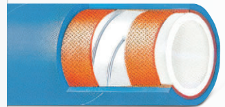
GIDA ALICI-VERİCİ HORTUM
